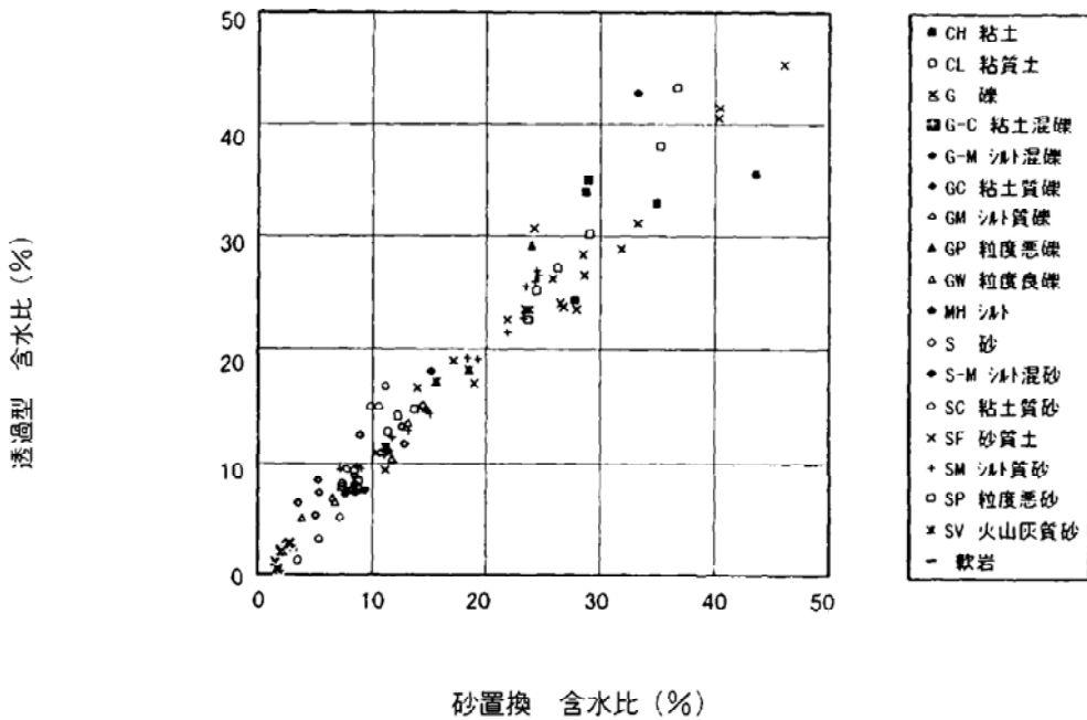
図-8 砂置換と透過型の相関 (含水比・土質別データ)
