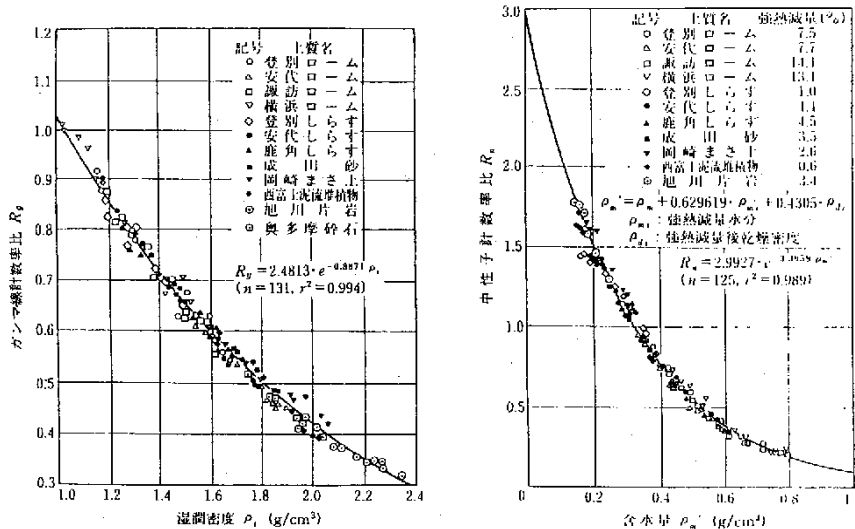
図-2 計数率比 (R) と密度および含水量の関係
