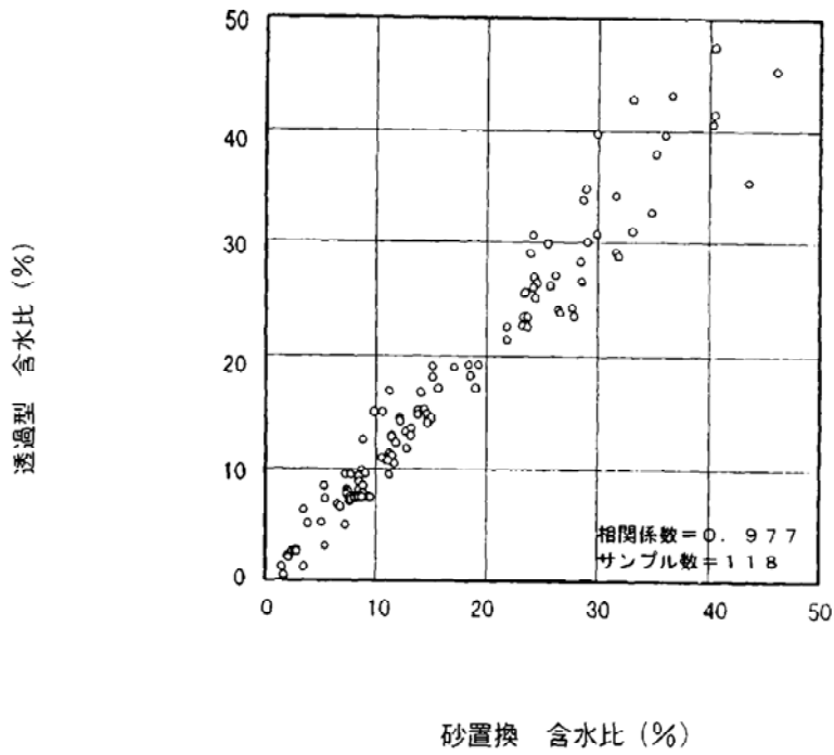
図-7 砂置換と透過型の相関 (含水比・全データ)
